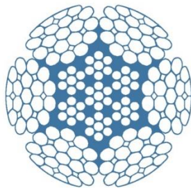
6x25F+IWRC
