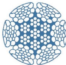
6x26SW+IWRC
