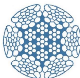
6x26SW+IWRC
